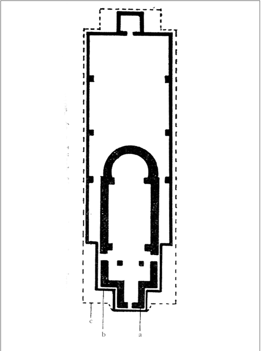
Mayerhoffer- és a Lösch-féle templom alaprajza: a – a régi templom; b – az első bővítés után; c – a mai alapterület
