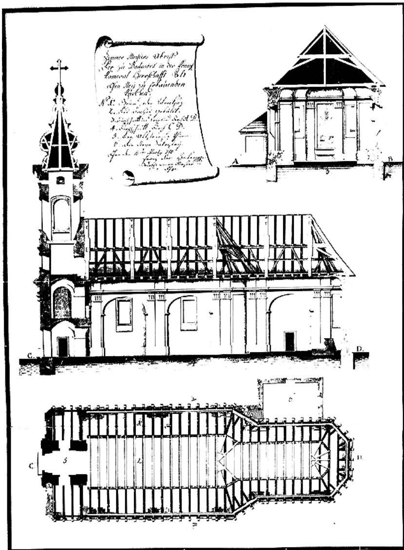
A királyi kamarai Óbudai uradalomban Budaörsön újonnan építendő templom ácsmesteri alaprajza 1780-ból
